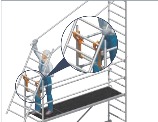
1. Aufstecken der ersten Standleiter. Anbringen der Uni Montagehaken und Positionierung der zweiten Standleiter zur Montage der Geländer.
